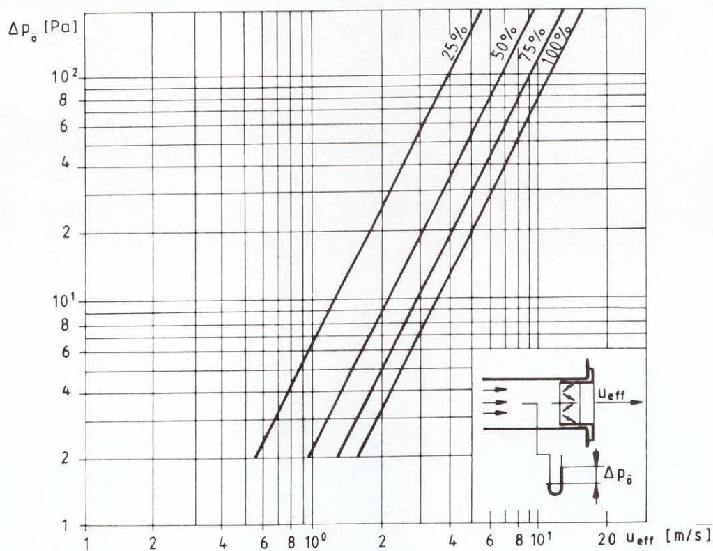
2. ábra AZ A2 típusjelű szabályozó zsalu szabályozási görbéi
