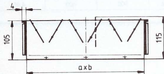
1. ábra AZC típusjelű szabályozó zsalu csavarkötéssel szerelhető szellőzőrácsokhoz
