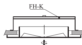
Álmennyezeti felszerelés FH-K híddal
