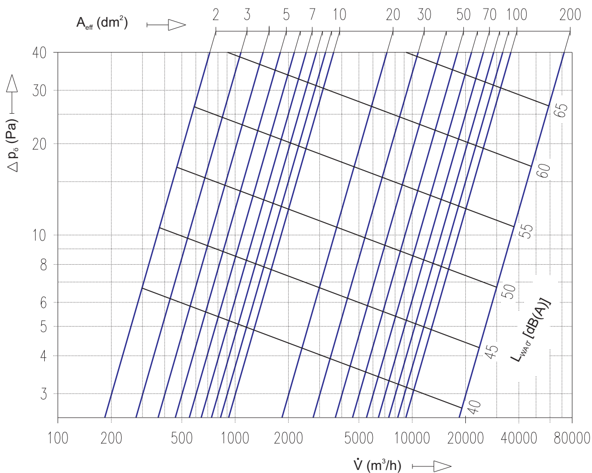
1.61-1 diagram USZ-17 zsáluk kiválasztása
